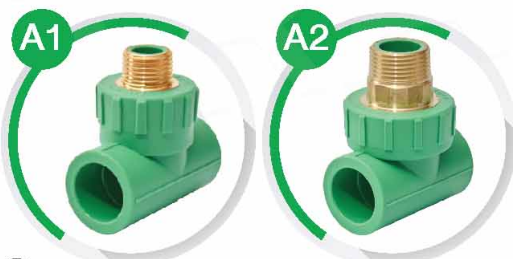
สามทางเกลียวนอกทองเหลือง พีพีอาร์ PP-R BRASS MALE TEE
