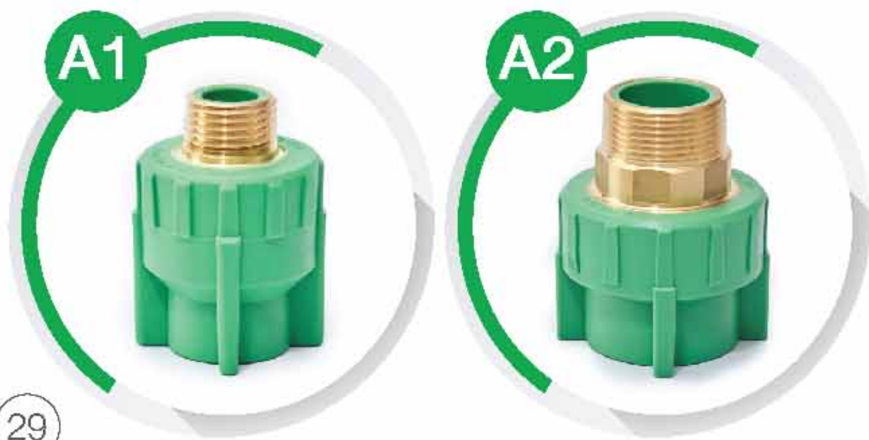
ข้อต่อตรงเกลียวนอกทองเหลือง พีพีอาร์ PP-R BRASS MALE SOCKET
